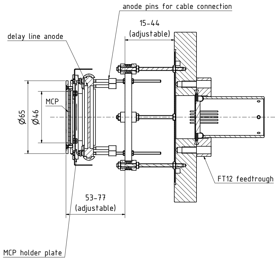
A-A ( 1 : 1 )
