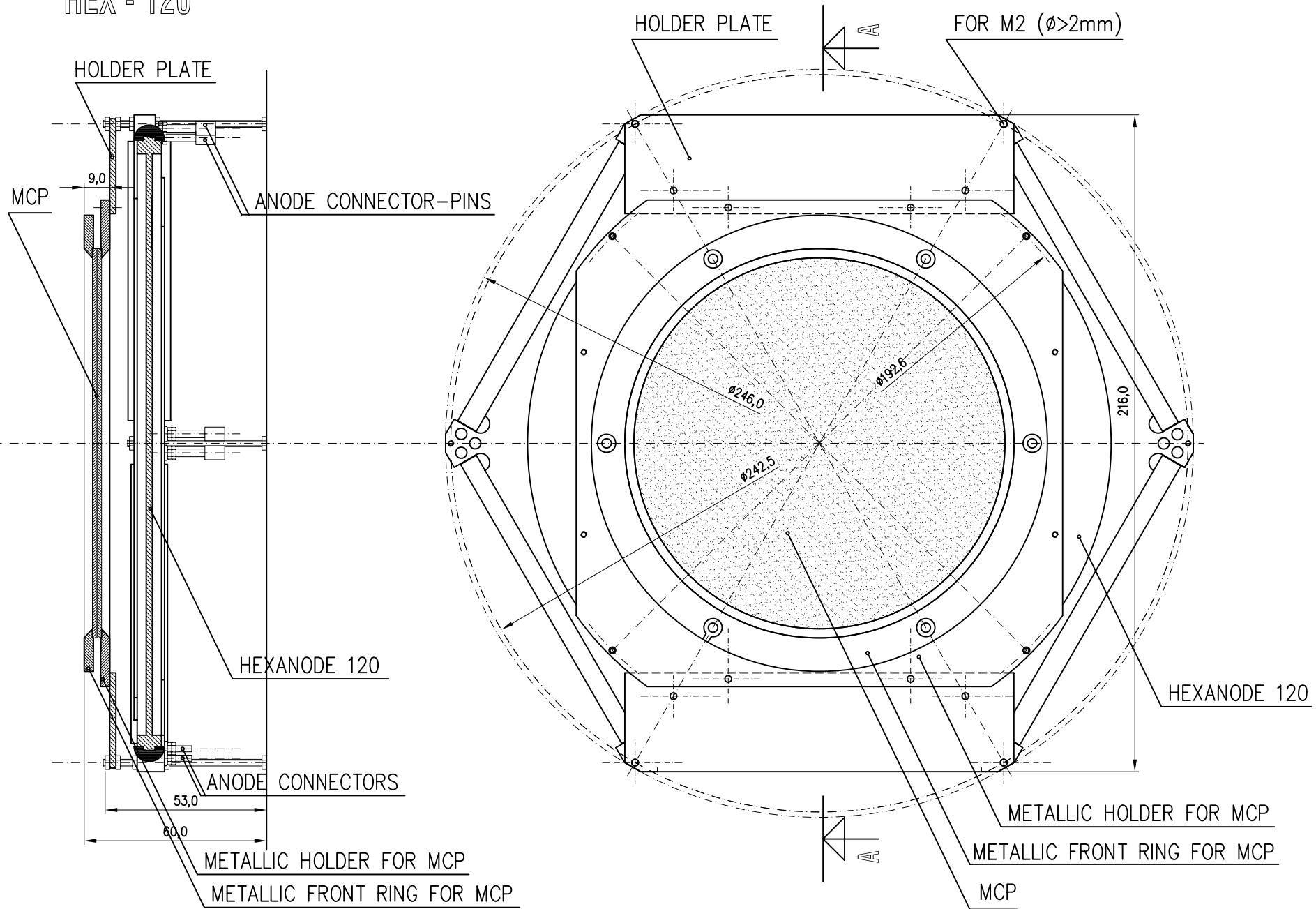
SECTION A-A
